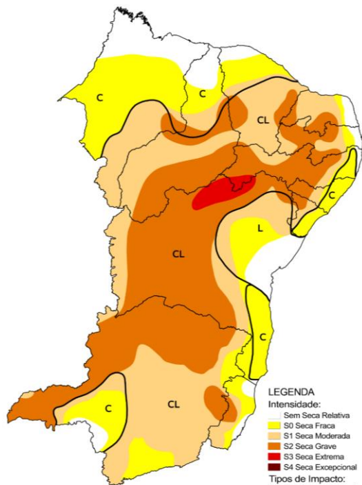
Monitor de Secas Novembro/2019
