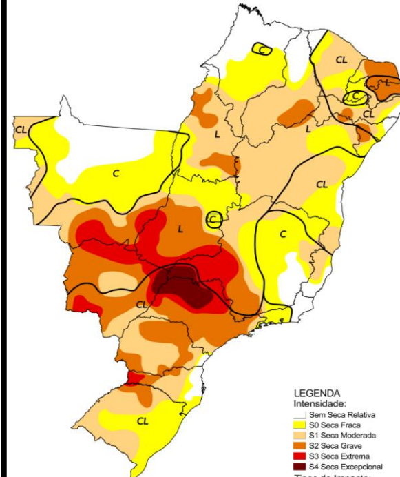
Monitor de Secas Novembro/2021
