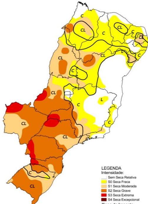
Monitor de Secas Novembro/2020
