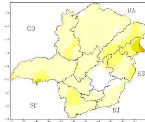
Anomalia período chuvoso 2017/2018
