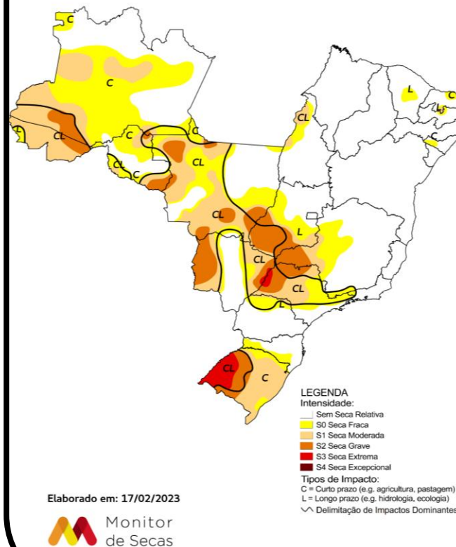
Monitor de Secas Janeiro/2023
