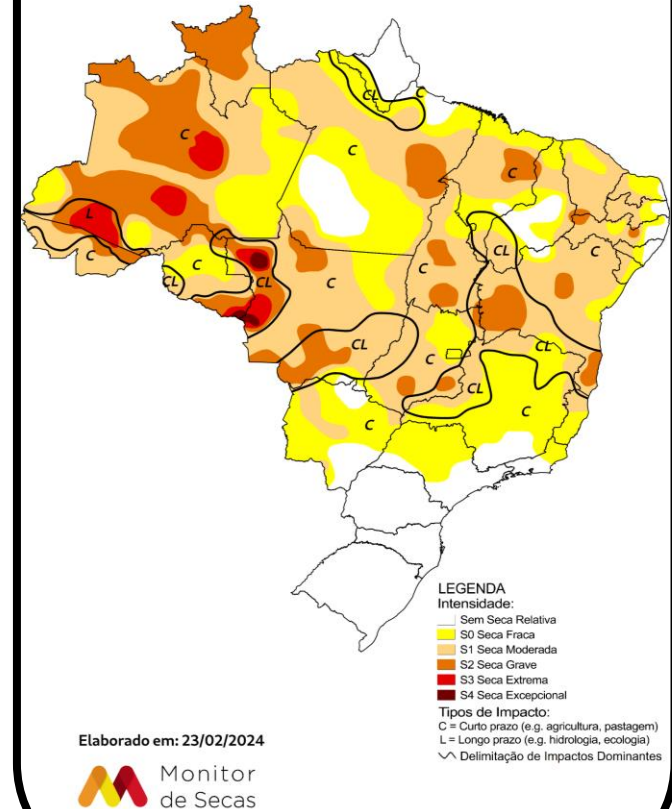
Monitor de Secas Janeiro/2024
