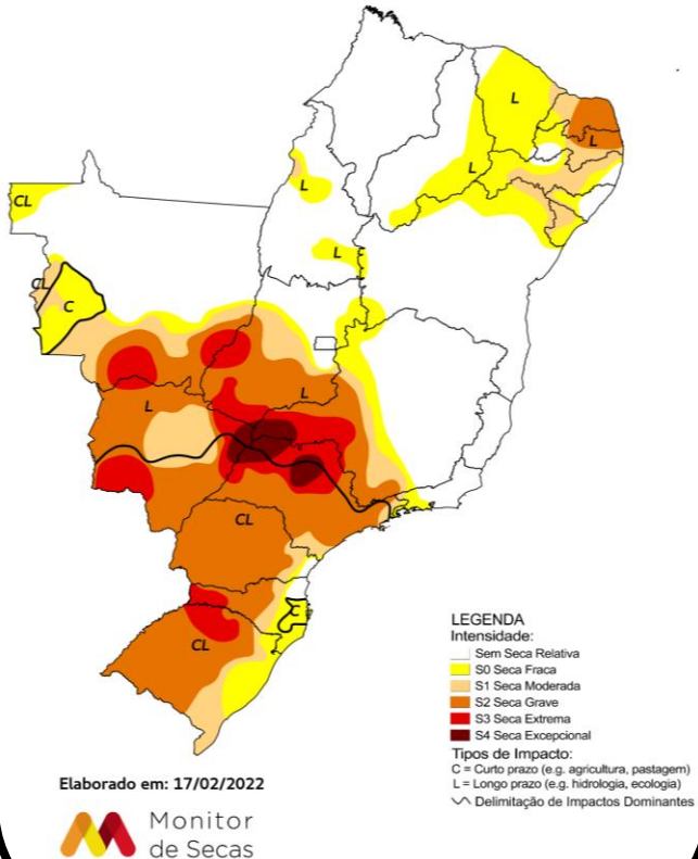
Monitor de Secas Janeiro/2022
